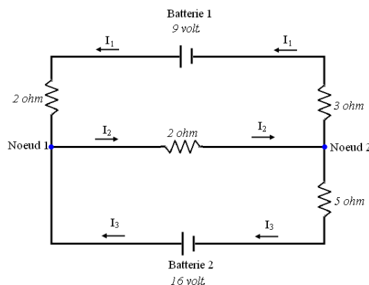
FIGURE 4.1 – Circuit électrique
