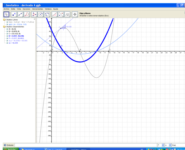
FIGURE 3.18 – Première ébauche de la fonction dérivée en considérant les pentes des tangentes.
