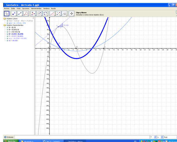
FIGURE 3.19 – Un dernier ajustement au coefficient quadratique pour que les deux courbées coïncident.
