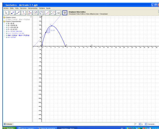
FIGURE 3.17 – Différentes représentations du même objet : une droite sécante à une fonction.
